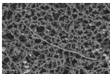
試料；白石綿 倍率；2,500倍
